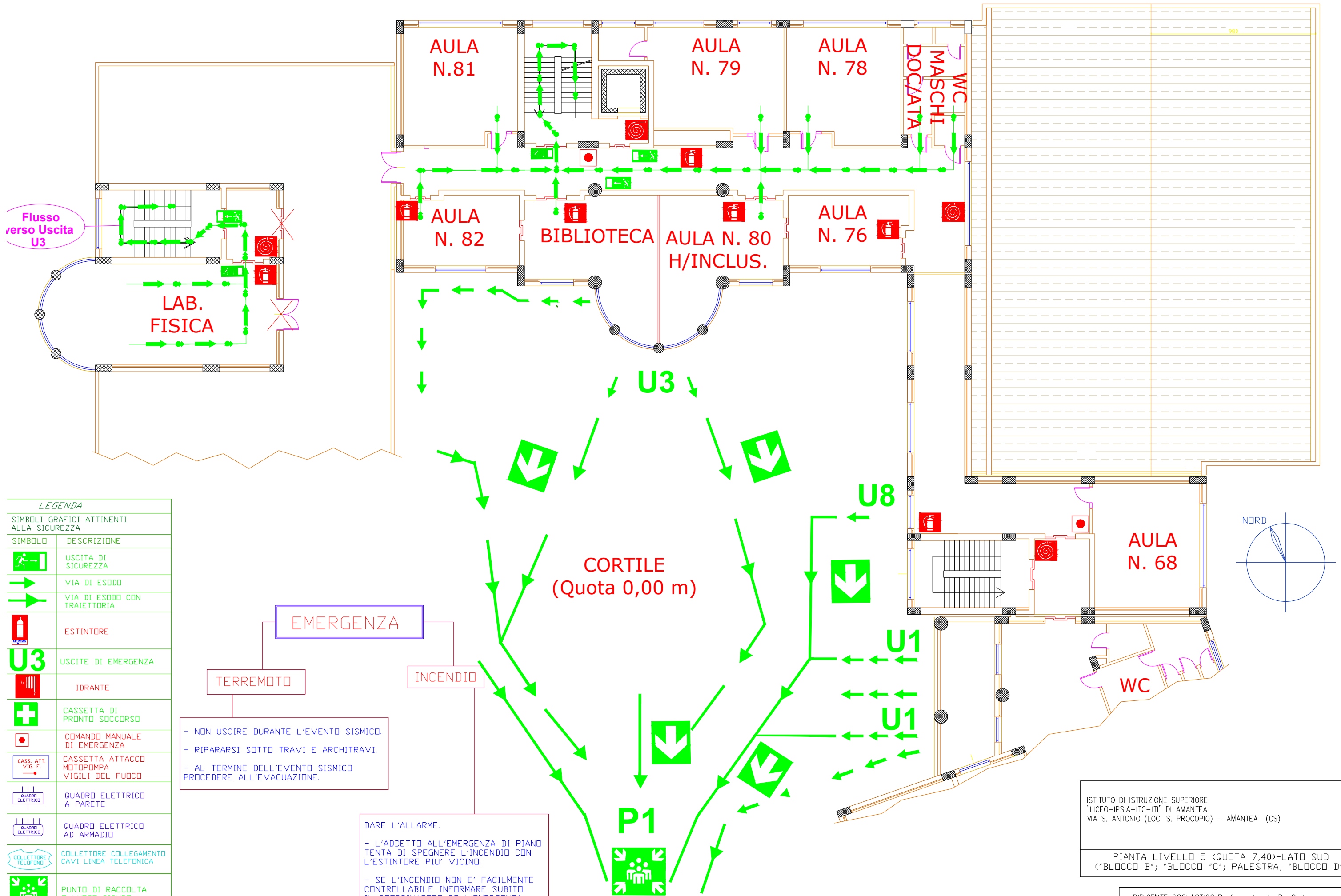
PIANTA DI EMERGENZA PIANO SECONDO
